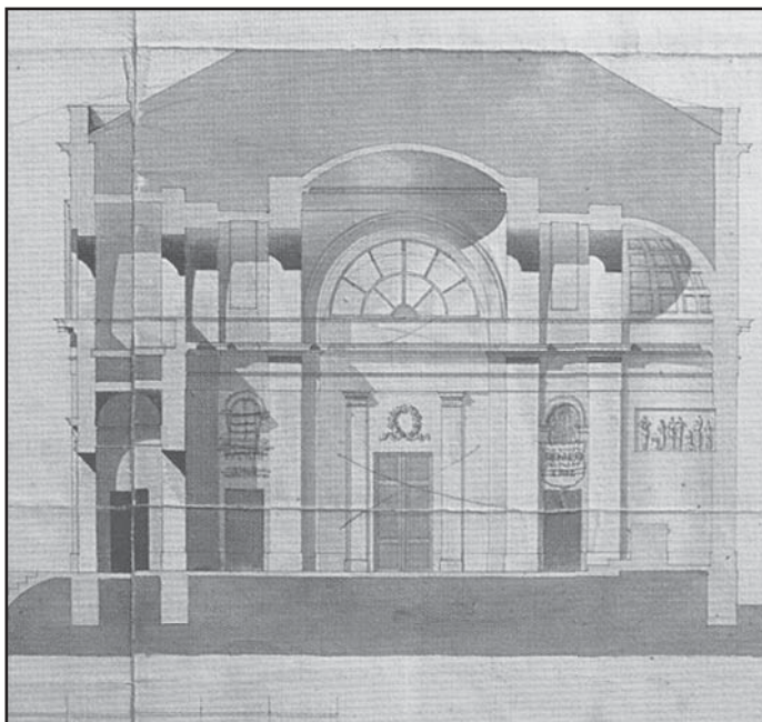
Původní návrh stavby kostela sv. Jana Nepomuckého v Hlohovci r. 1831 (podélný řez). Lednicko-Valtický areál, Průvodce.
